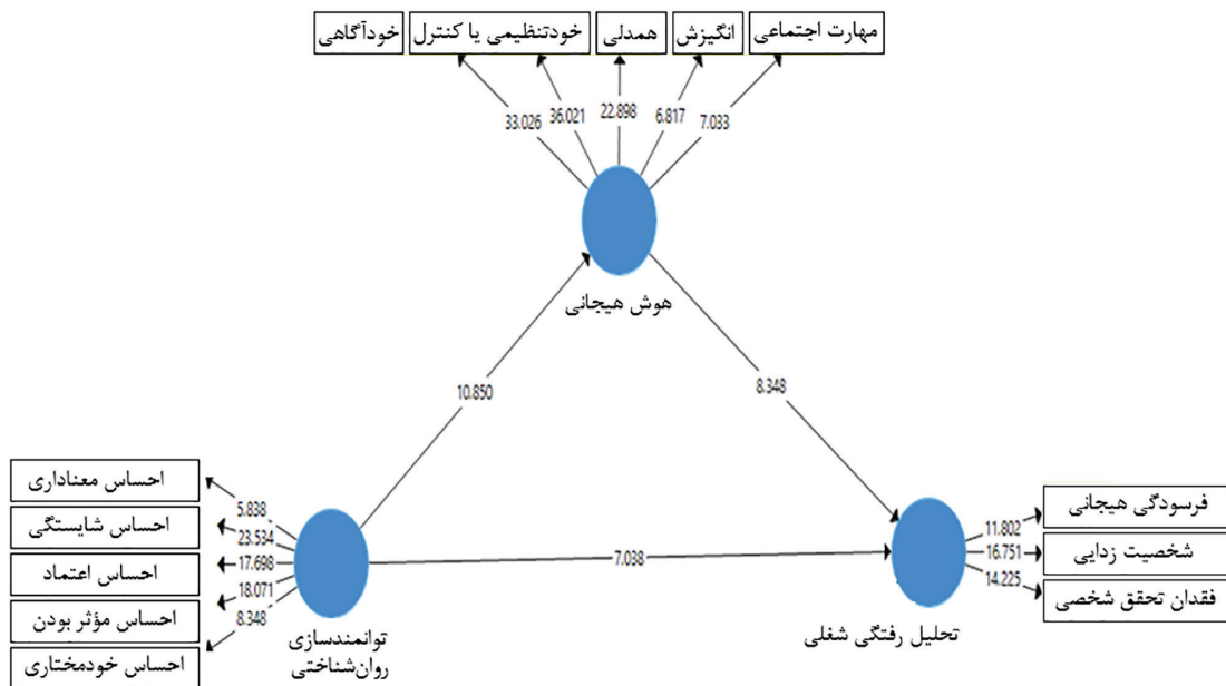
شکل ۲. آماره تی بوت استرپینگ مدل تحقیق (مدل بیرونی تحقیق)
