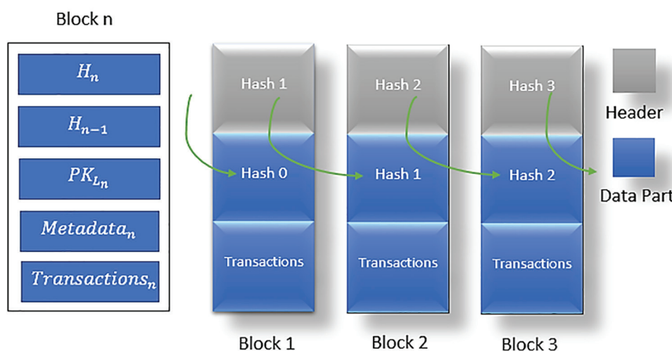
شکل ۲. تابع هش و ساختار بلوکی اطلاعات در سیستم فناوری زنجیره بلوکی پسارزیابی وسایل پزشکی
